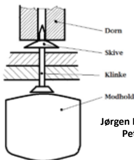
1,8 mm kobbersøm Simpson Construction tætningsmasse
